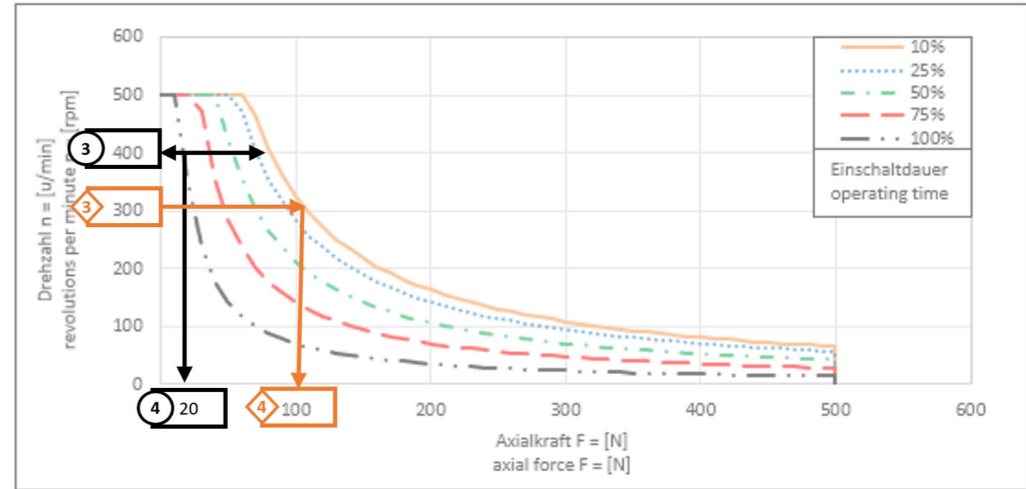
Ablesebeispiel Diagramm 2: Axialkraft / Drehzahl
